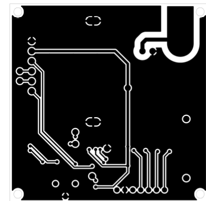
CDP-RX-03AS-TestNew 16680
